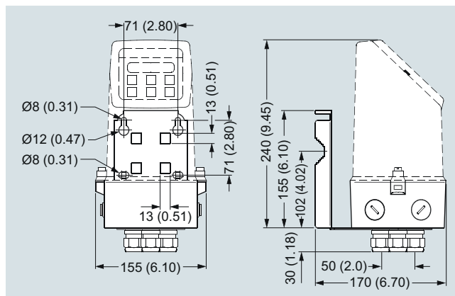
Transmetteur, montage mural, dimensions en mm (inch)
