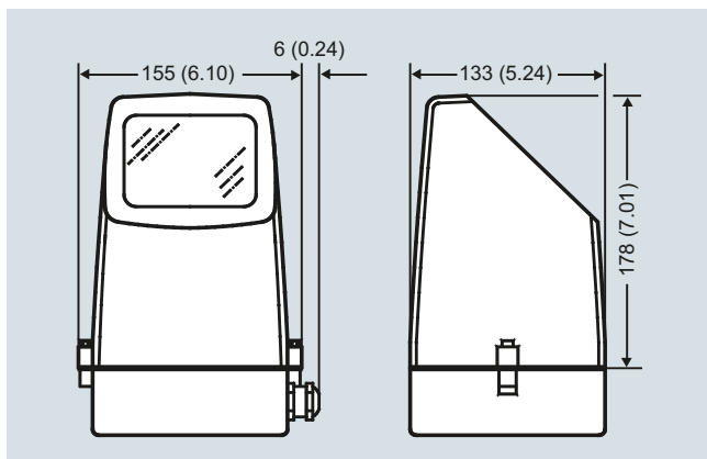
Transmetteur, montage compact, dimensions en mm (inch)
